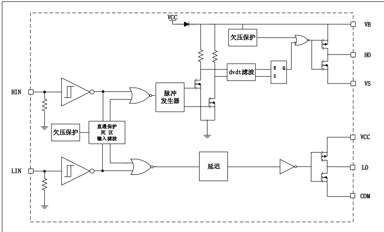
图 4: TR2302内部功能图
