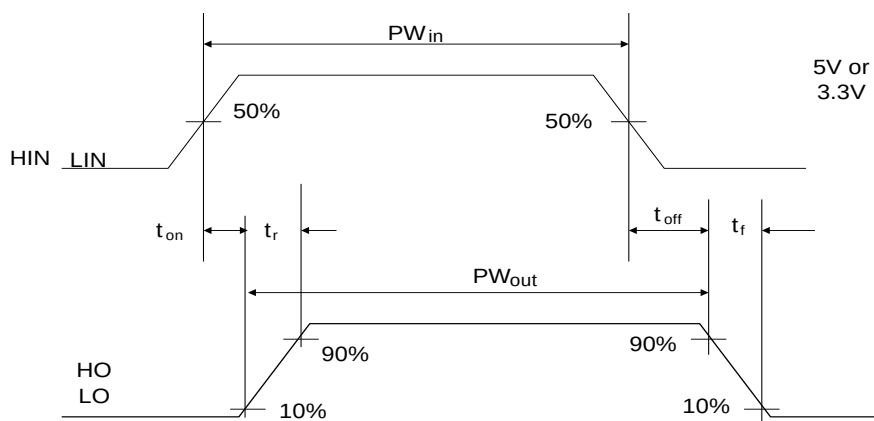
图2: TR2302 传输时序图
