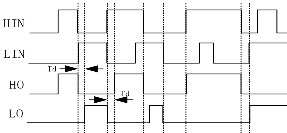
图2: TR2302 传输时序图
