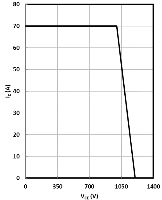
Fig. 6 RBSOA
