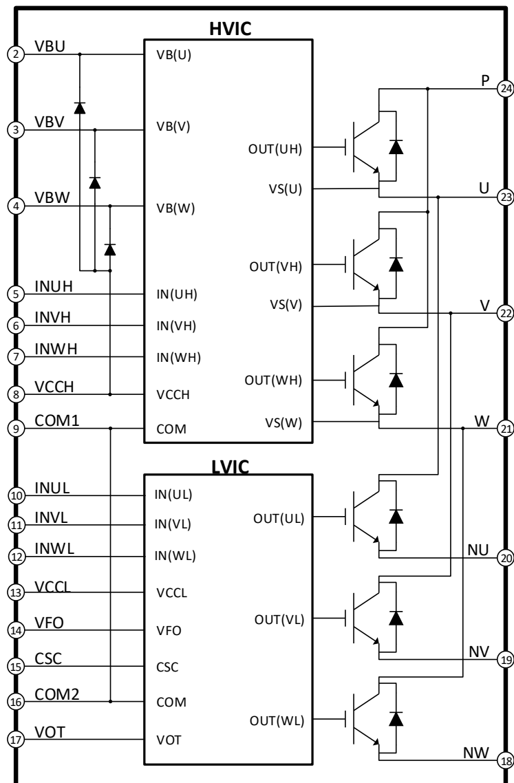
图 1 DPM30C60 功能框图
