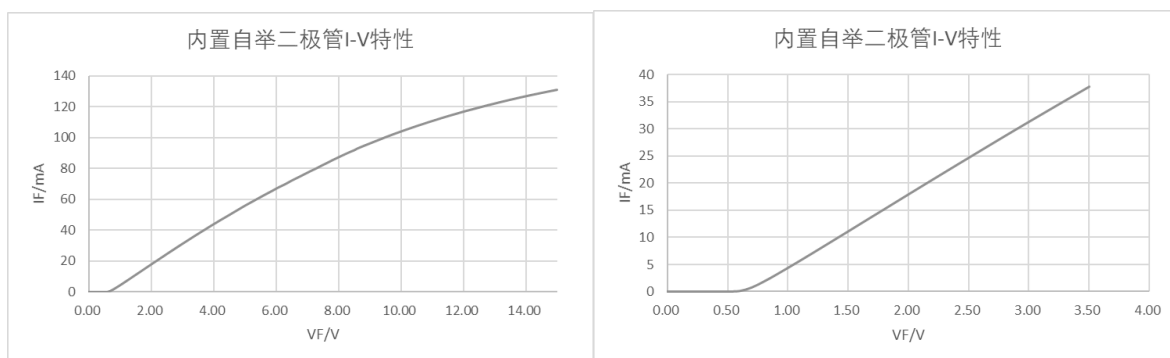
图 4 内置自举二极管特性曲线
