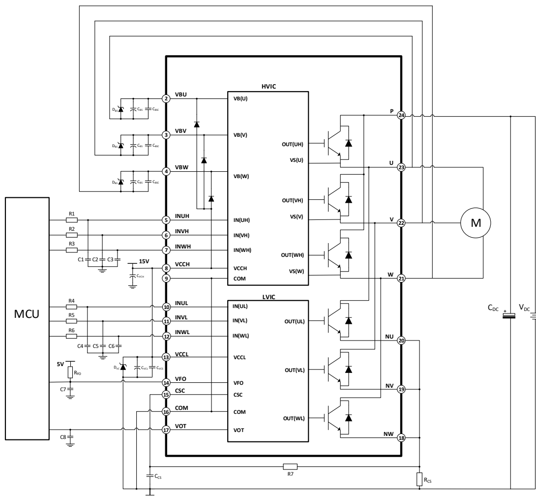
图 10 DPM30C60 典型应用线路
