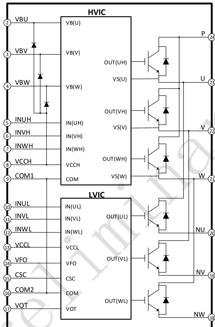
图 1 DPM20C60DG 功能框图
