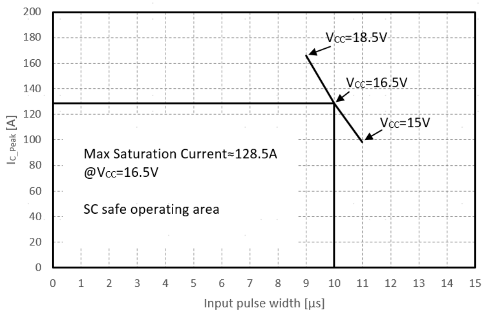
图 6 短路安全工作区
