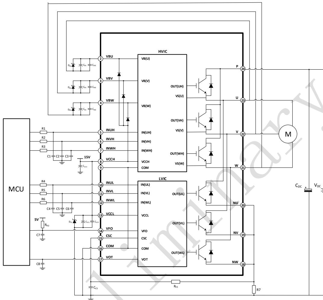
图 11 DPM20C60DG 典型应用线路
