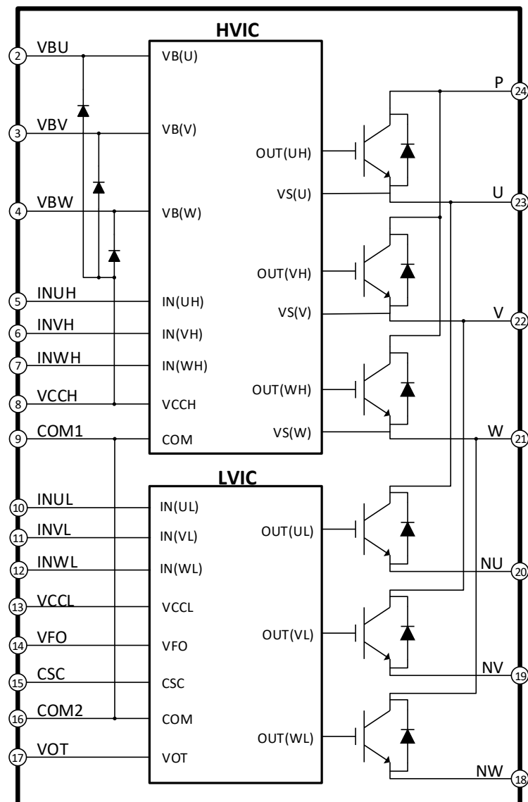
图 1 DPM20C60 功能框图
