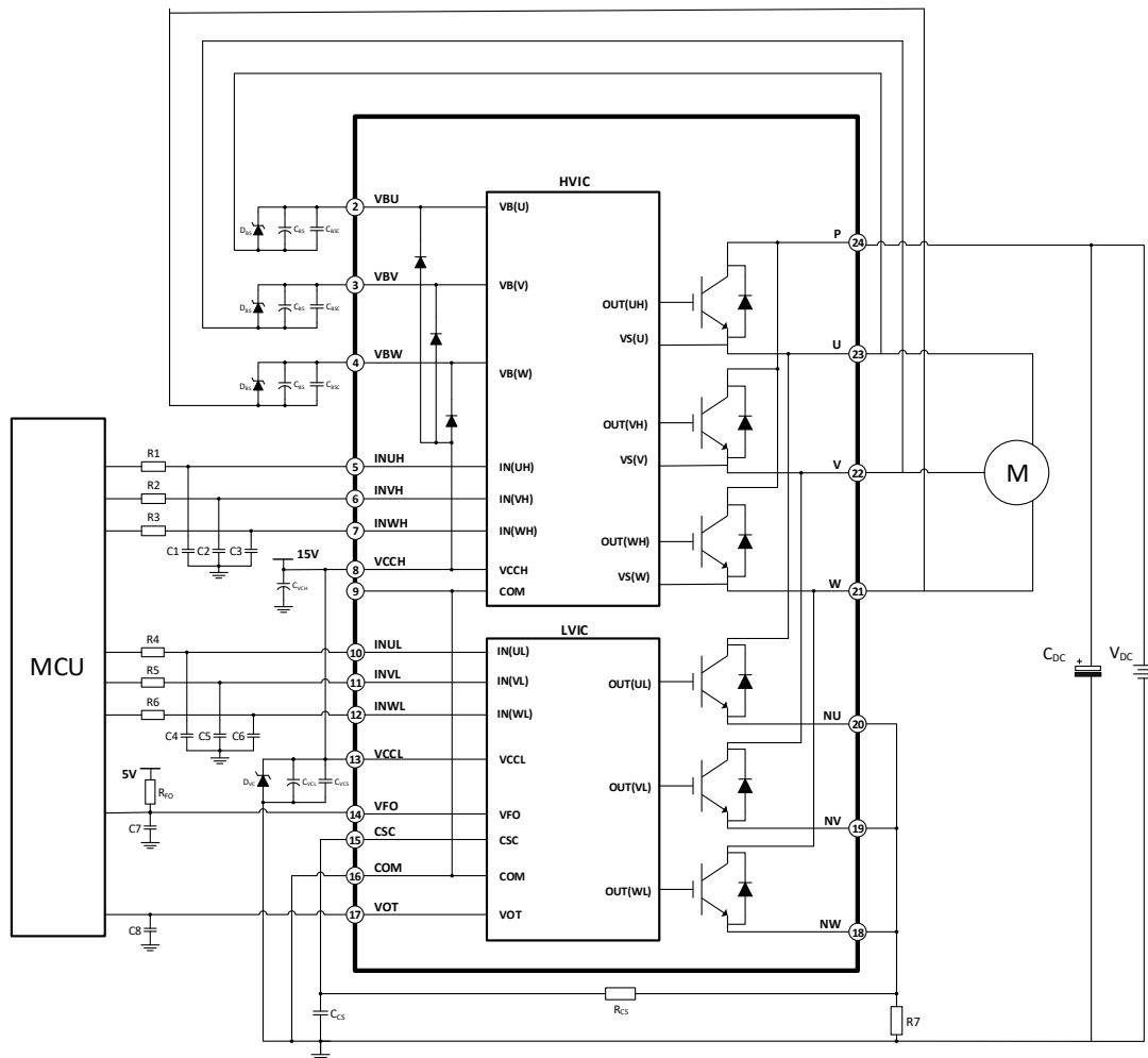
图 11 DPM20C60 典型应用线路
