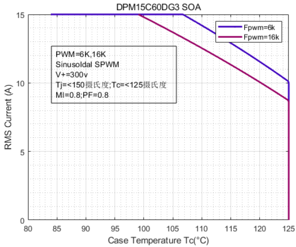
图 6 安全工作区（SOA 曲线）
