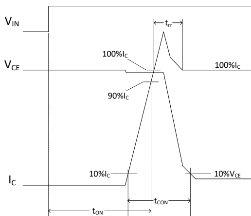
(1) 开通时间定义
