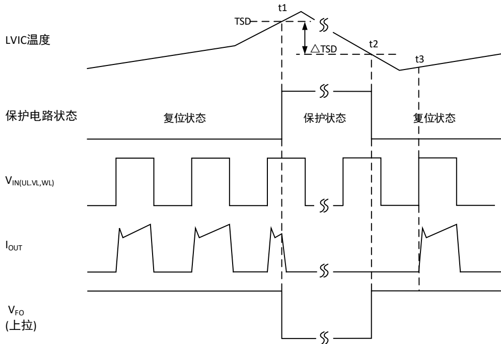
图 7 LVIC 过温保护功能时序图
