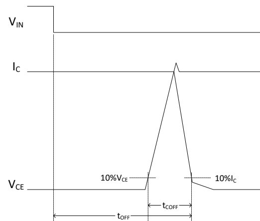
(2) 关断时间定义
