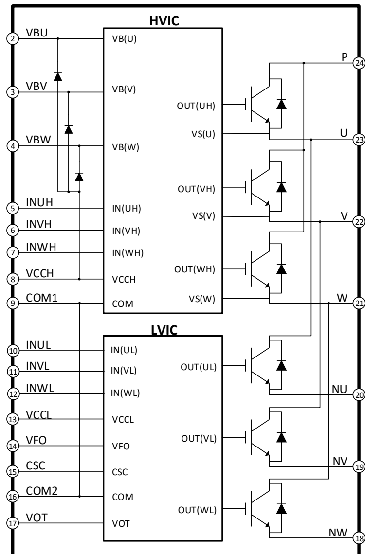
图 1 DPM10C60DG 功能框图
