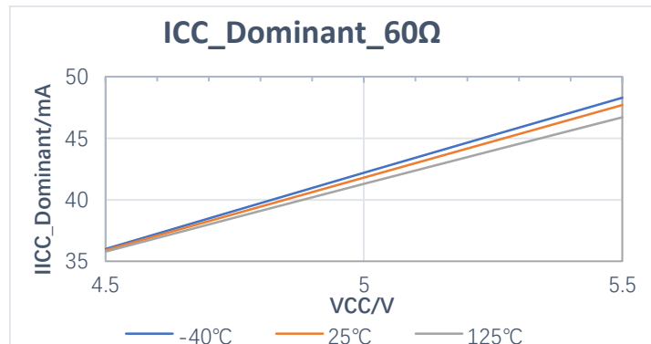
图 9-4 60Ω 负载下显性状态电流
