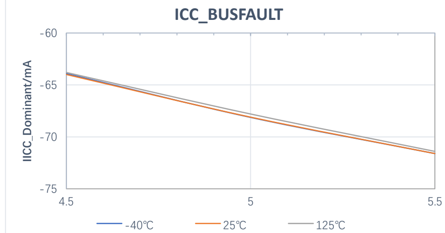
图 9-5 BusFault 电流
