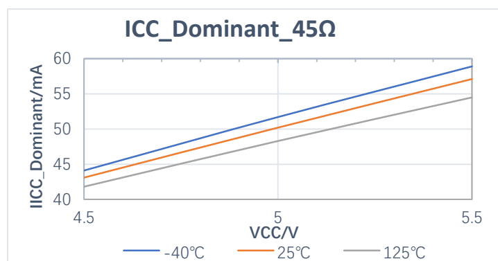
图 9-3 45Ω 负载下显性状态电流
