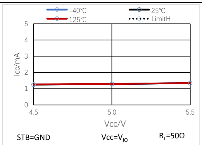
图 8-2 隐性状态 I_{cc} 电流
