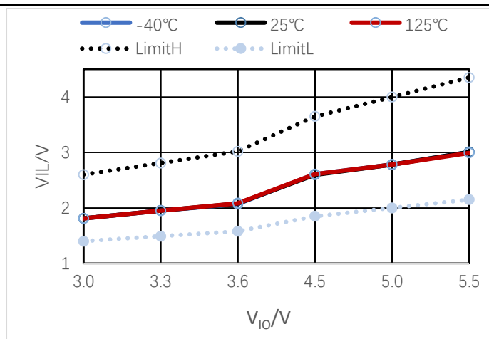
图 8-8 STB 管脚逻辑低电平
