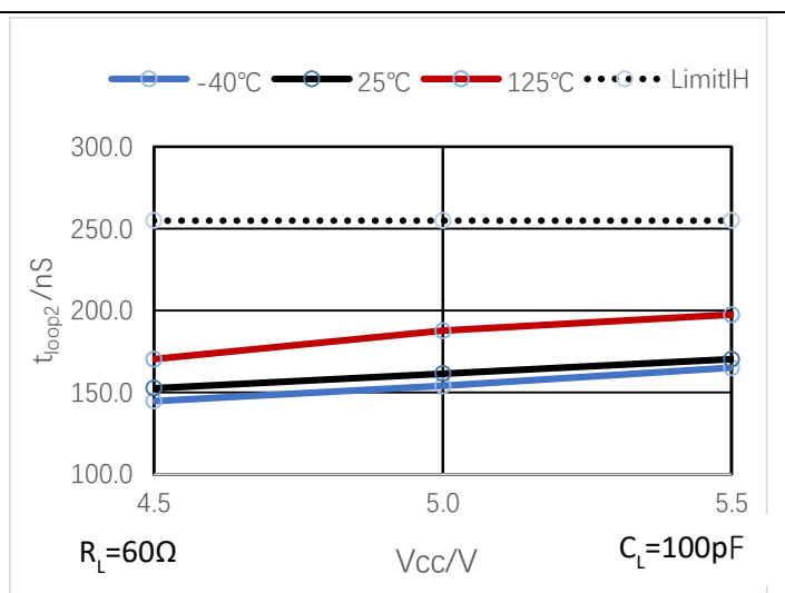
图 8-16 Loop2 Delay
